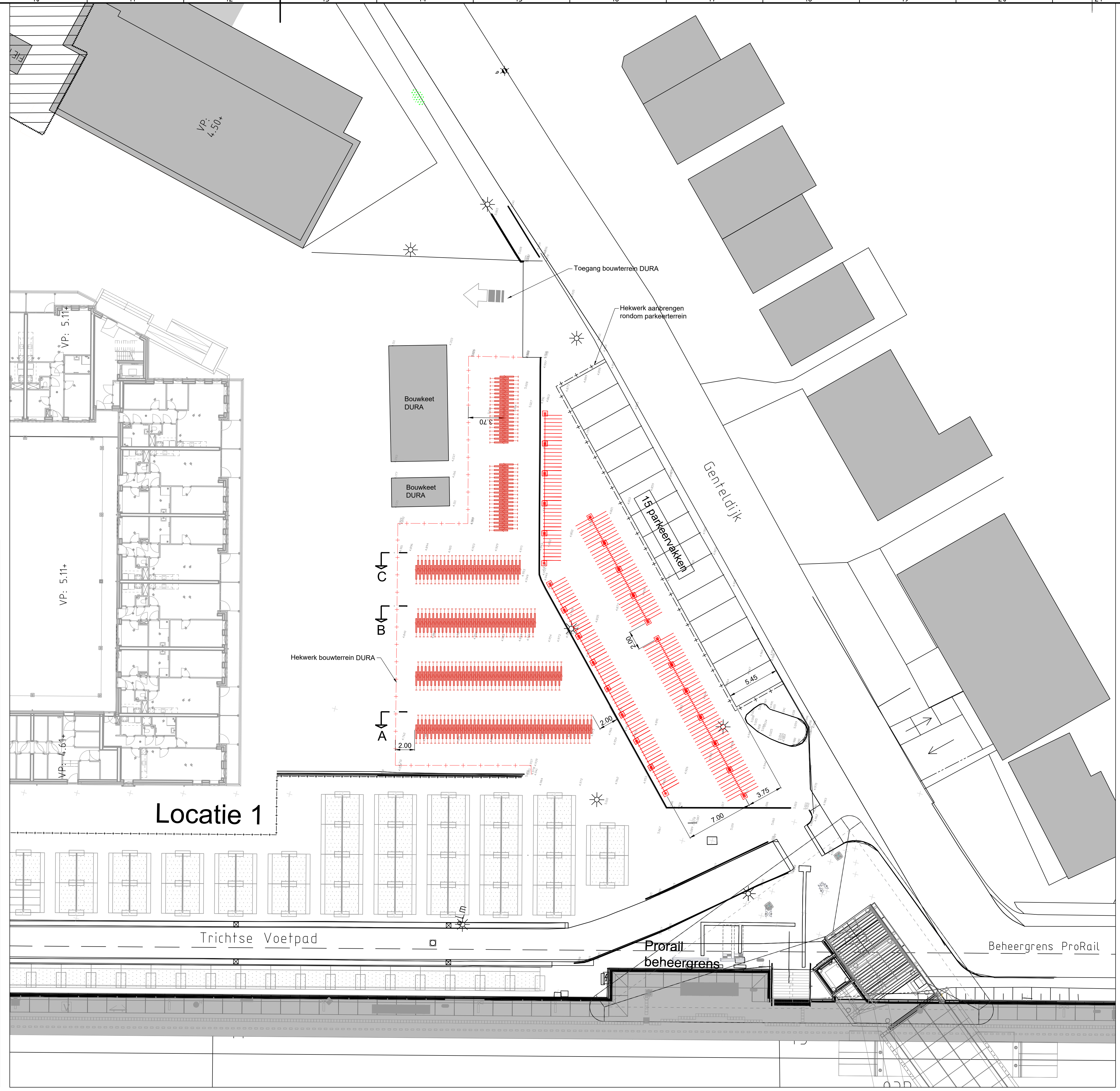
Plattegrond tijdelijke stalling, locatie 1 | schal 1:200
