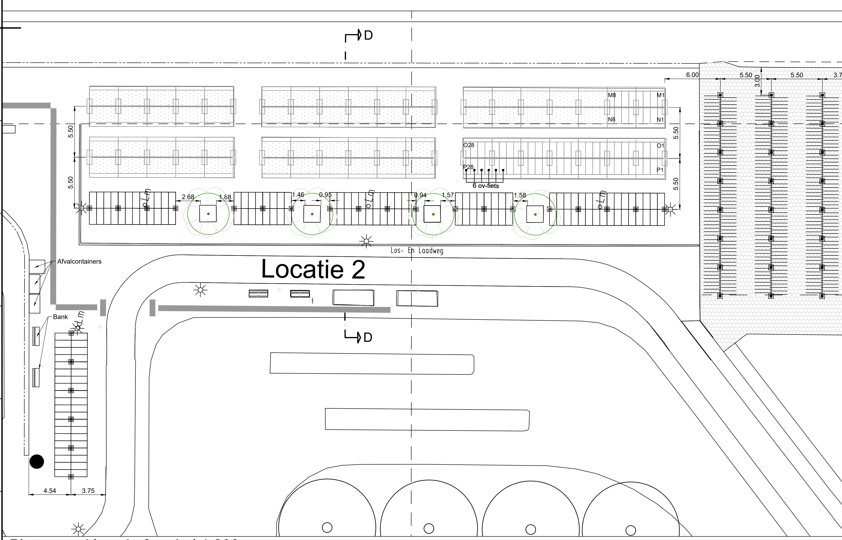
Plattegrond locatie 2, schal 1:200
