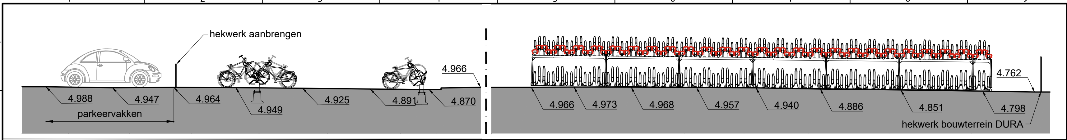
Doorsnede A, tijdelijke stalling, schal 1:100
