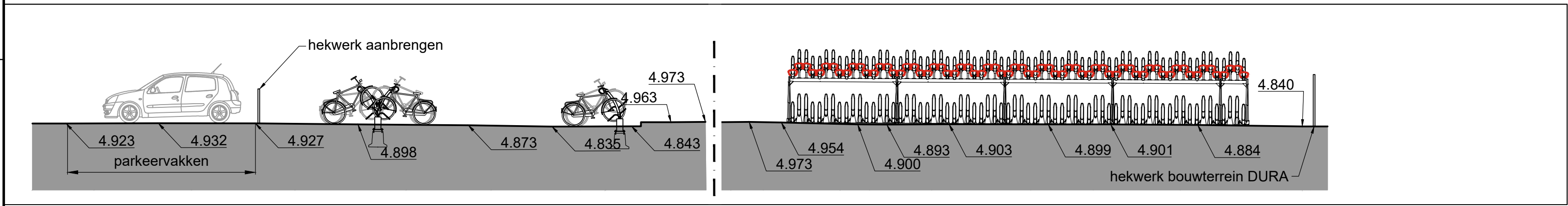
Doorsnede B, tijdelijke stalling, schal 1:100
